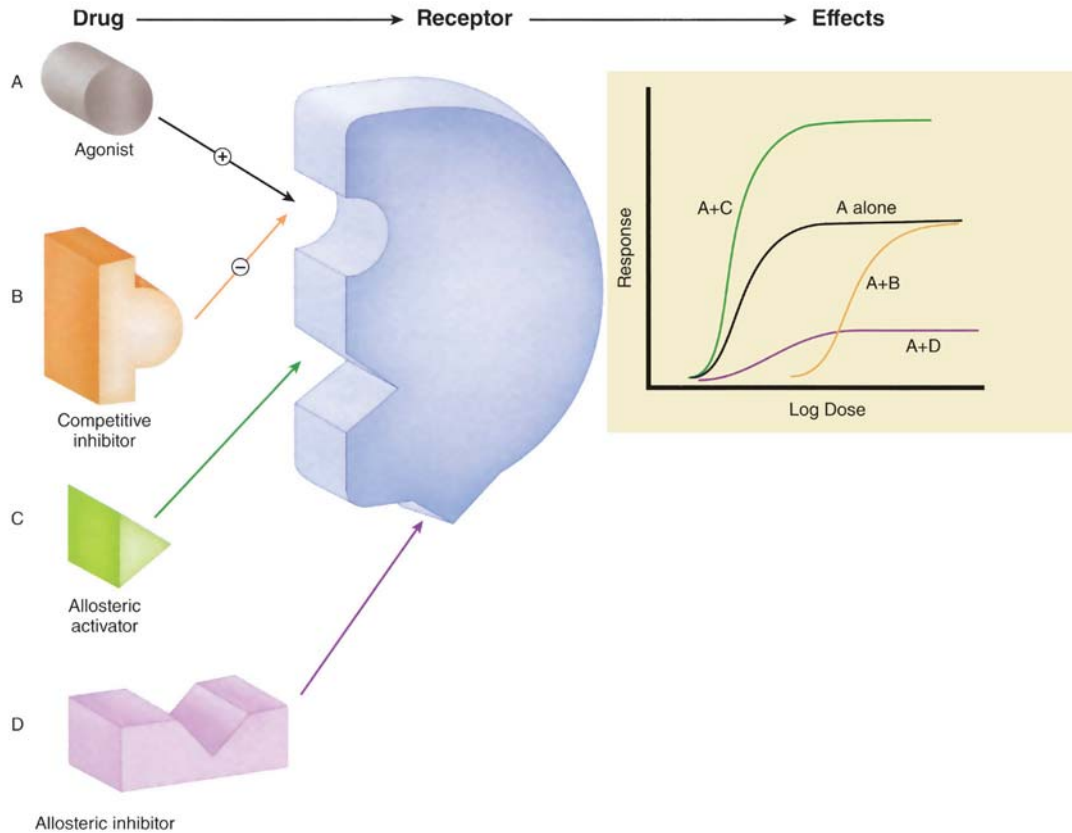
شکل ۲-۱. داروها از راه‌های متعددی با گیرنده‌ها تعامل می‌کنند. اثرات حاصل از این تعامل‌ها، در منحنی‌های مقدار مصرف پاسخ در سمت راست شکل نشان داده شده‌اند. داروهایی که پاسخ آگونیست (A) را تغییر می‌دهند، ممکن است در جایگاه اتصال آگونیست عمل کنند و با آگونیست رقابت نمایند (مهارکننده‌های رقابتی، B)، و یا این که در جایگاه‌های مجزایی اثر کنند (آلوستریک) و پاسخ به آگونیست را افزایش (C) یا کاهش (D) دهند. فعال‌کننده‌های آلوستریک (C) ممکن است کارایی آگونیست یا میل اتصال آن را افزایش دهند. این منحنی، افزایش کارایی را نشان می‌دهد، افزایش میل اتصالات سبب جایجایی منحنی به طرف چپ می‌شود.
