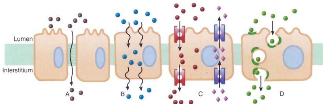
شکل ۴-۱. مکانیسم‌های نفوذ دارو. داروها ممکن است به صورت غیرفعال از طریق کانال‌های آبی موجود در پیوستگاه‌های بین سلولی (مثل اتصالات محکم، A) انتشار پیدا کنند، و یا از غشاهای لیپیدی سلول‌ها عبور نمایند (B). برخی داروها که خواص ویژه‌ای دارند، به وسیله حامل‌هایی به سلول‌ها وارد یا از آنها خارج می‌شوند (C). داروهای بسیار نفوذناپذیر نیز به گیرنده‌های سطح سلول متصل می‌شوند (جایگاه‌های اتصال سیاه‌رنگ)، به وسیله غشای سلول احاطه می‌شوند (آندوسیتوز)، و سپس به داخل سلول آزاد می‌شوند و یا به واسطه وزیکول‌های غشادار، به خارج از سلول و به فضای خارج سلولی رها می‌شوند (اگزوسیتوز، D).
